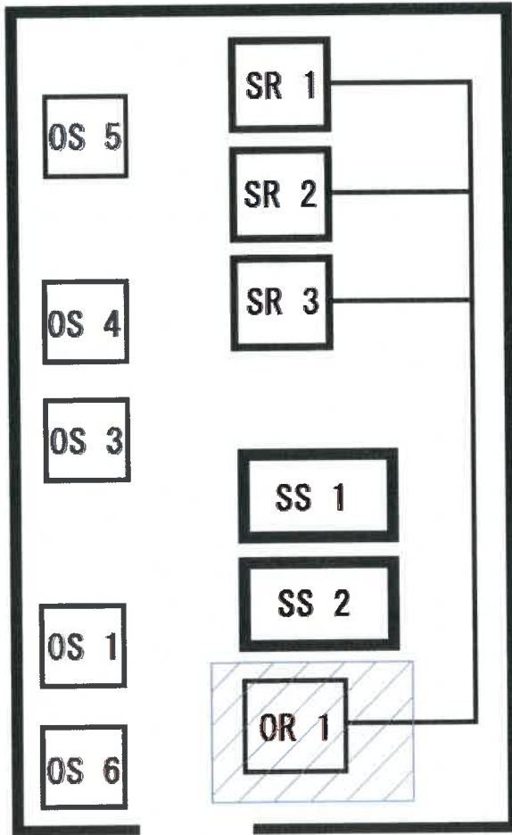
Rys1. Umieszczenie osuszacza OR 1 w budynku sprężarkowni.
