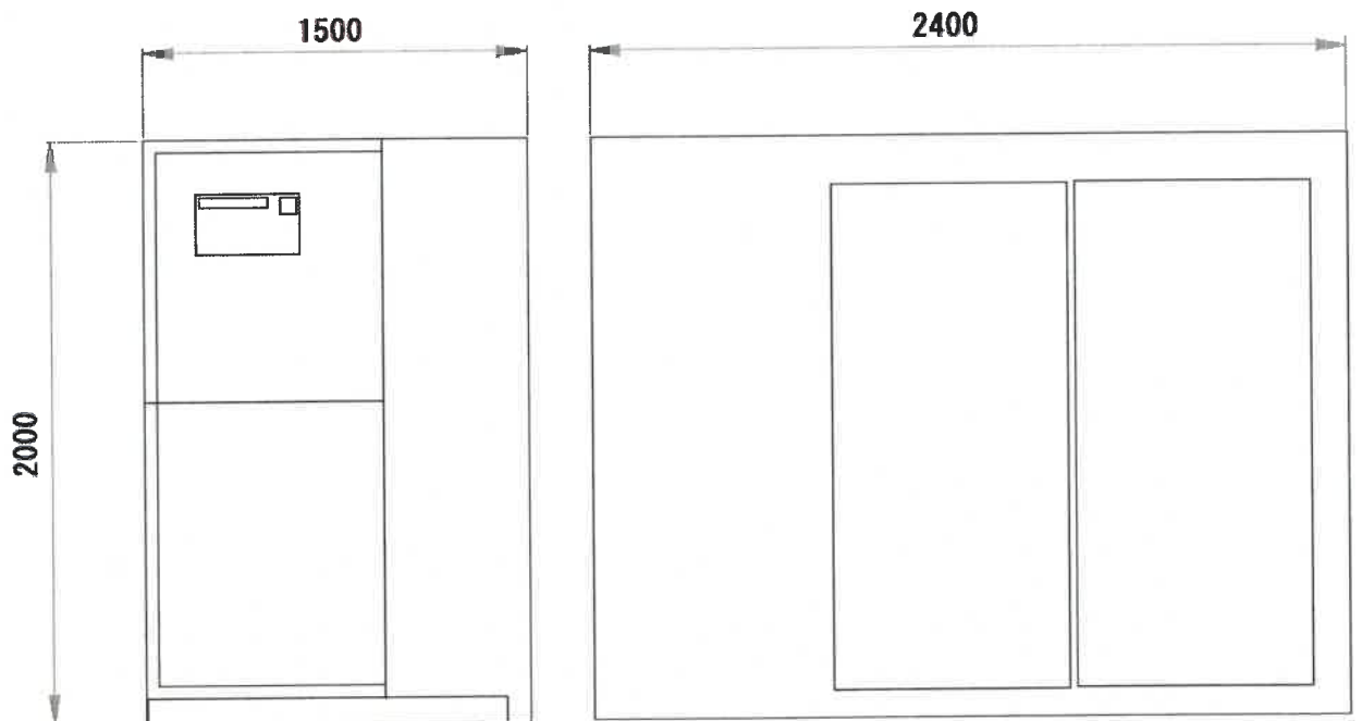
Rys2. Dopuszczalne wymiary (max) zamawianego osuszacza.
